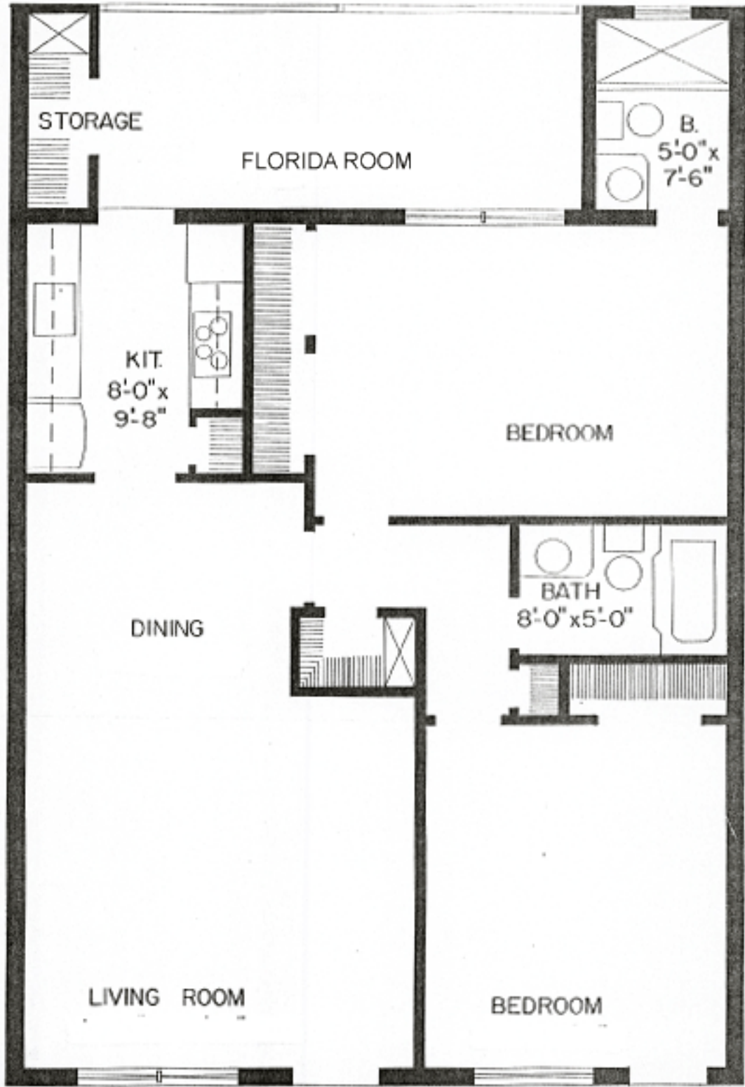
DELUXE - 2 BEDROOM - UP
